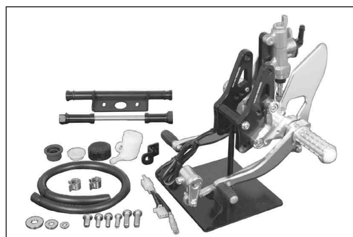
リアマスターシリンダー
