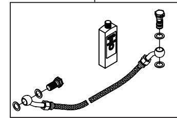
06-08-0095 リアブレーキホースキット (500mm)
