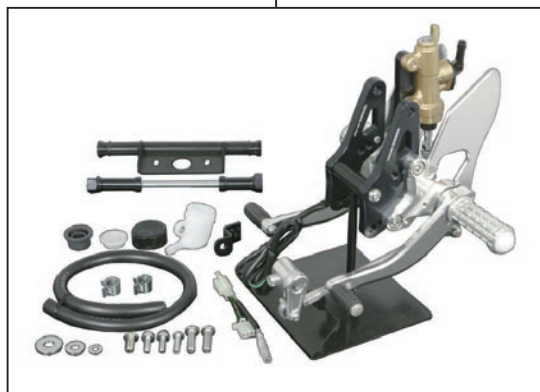
06-13-0010 バックステップキット (ディスク /3ポジション変更タイプ)
