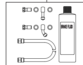
06-08-0097 リアブレーキホースキット (500mm)
