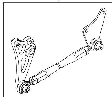
00-06-0044 リアキャリパーブラケットキット (フローティングタイプ)
