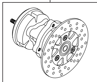
06-08-0025 リアディスクハブキット (ダンパー、タイプ2)
