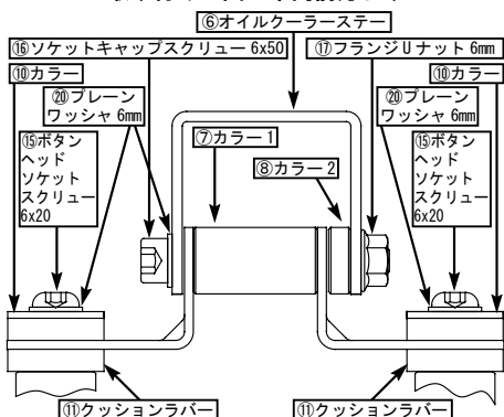
取り付けの図 車両前方より
