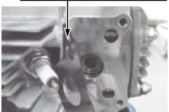
R. シリンダーヘッドカバーガスケット
