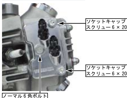
ノーマル6角ボルト
