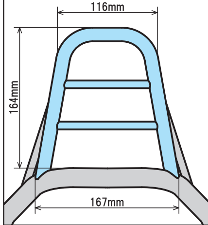
リアキャリア詳細図
