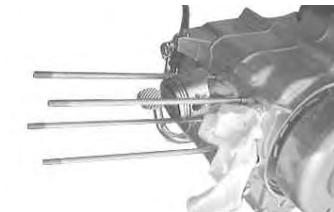
クランクケースのシリンダーホールとカムチェーン部にゴミや部品などを絶対落とさないようにウエスを詰め込む。
