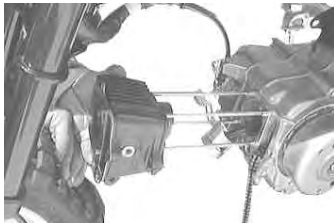
ピストンが抜けたらタイヤを手で押さえながらシリンダーを前方へ取り外す。
