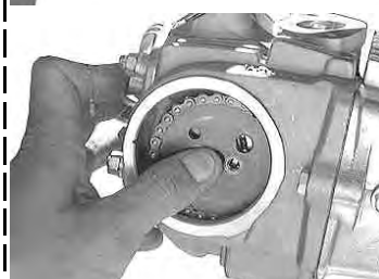
バルブクリアランス (インテーク側)
