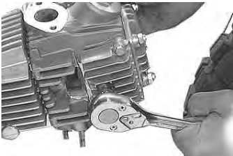
シリンダーヘッド右側の六角ボルト(矢印)を締める。
