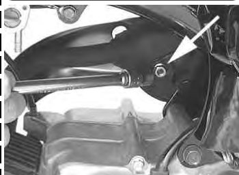
マフラー本体裏側にナットを取り付ける。(仮止め)
