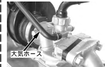
フューエルホースと大気ホースを取り付ける。
