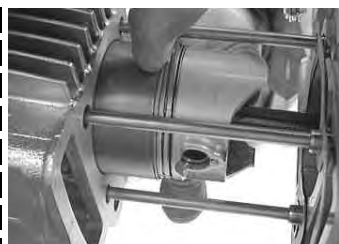
シリンダーをピストンリングの合い口がずれないようにしながら指で押し少しずつはめる。
