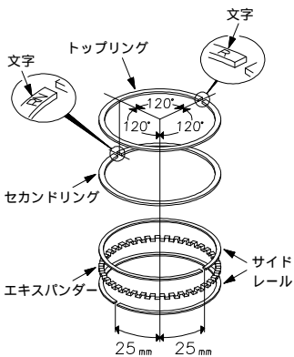
セカンドリングを入れる。
