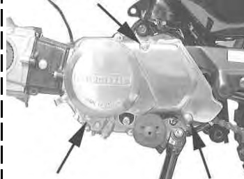
クランクケース左カバーを止めているボルト3本を取り付ける。
