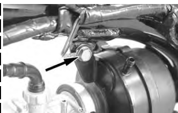
エアクリーナーステー部のボルトをアース線と共締めで取り付ける。
